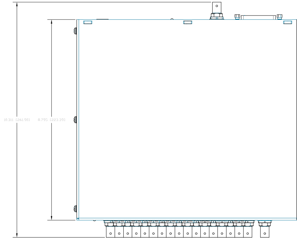
DT9857E-16
